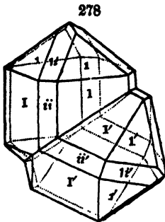
Cassiterite.
